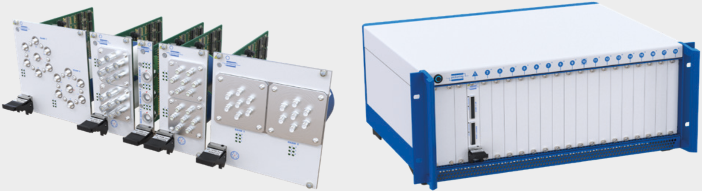
그림 1 - PXI 모듈 및 PXI 채시의 범위
